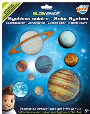
2013DF10 (6) Glow-in-the-dark Solar System | Système Solaire
